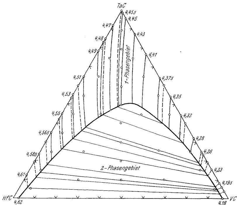
Abb. 4. HfC—VC—TaC; Schnitt bei 2050° C. Gitterkonstanten in Ångström
