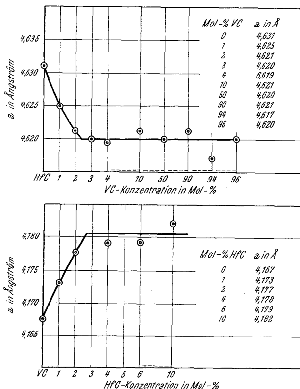
Abb. 1. Verlauf der Gitterkonstanten von HfC in Abhängigkeit von der VC-Konzentration bei 2050°C
