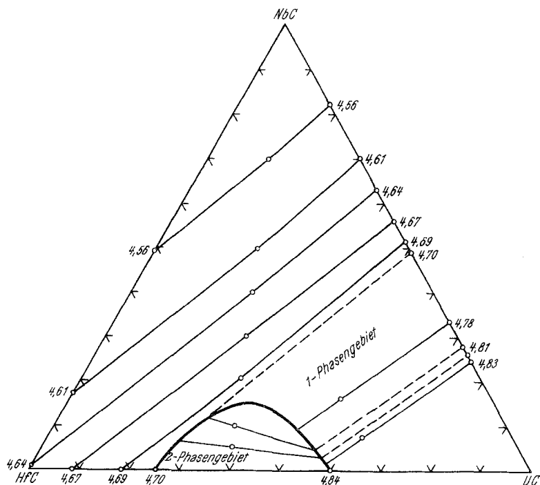
Abb. 6. HfC—UC—NbC: Schnitt bei 2050° C. Gitterkonstanten in Ångström
