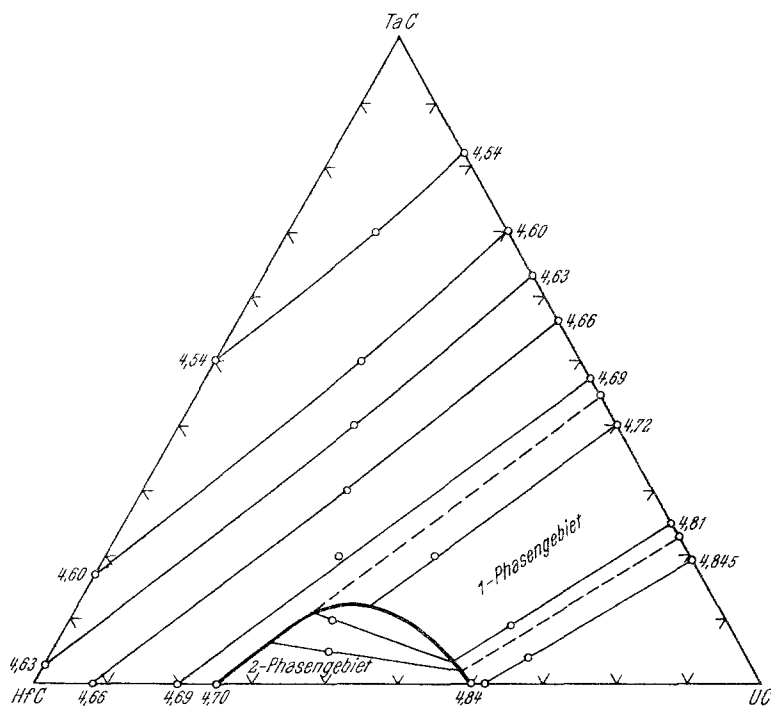
Abb. 7. HfC—UC—TaC: Schnitt bei 2050° C. Gitterkonstanten in Ångström
